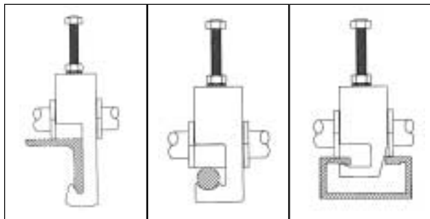
Angle KwikClamp
