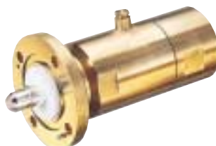
1-5/8" EIA Flange 87G
